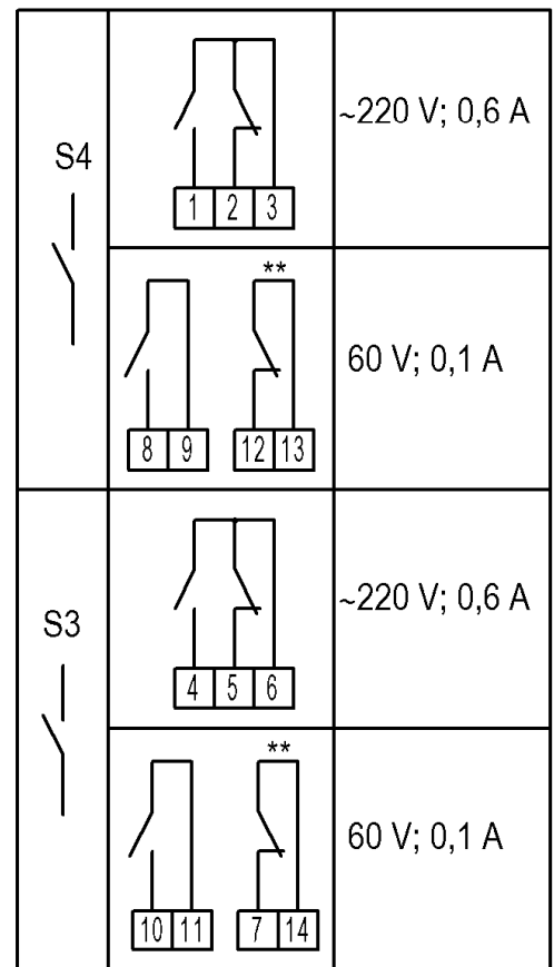
Рис.Б.4 - Схема подключений блока питания при использовании микровыключателей S3, S4 блока датчика
