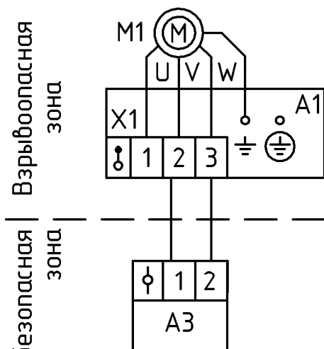
Рис.Б.1 - Схема электрическая принципиальная
