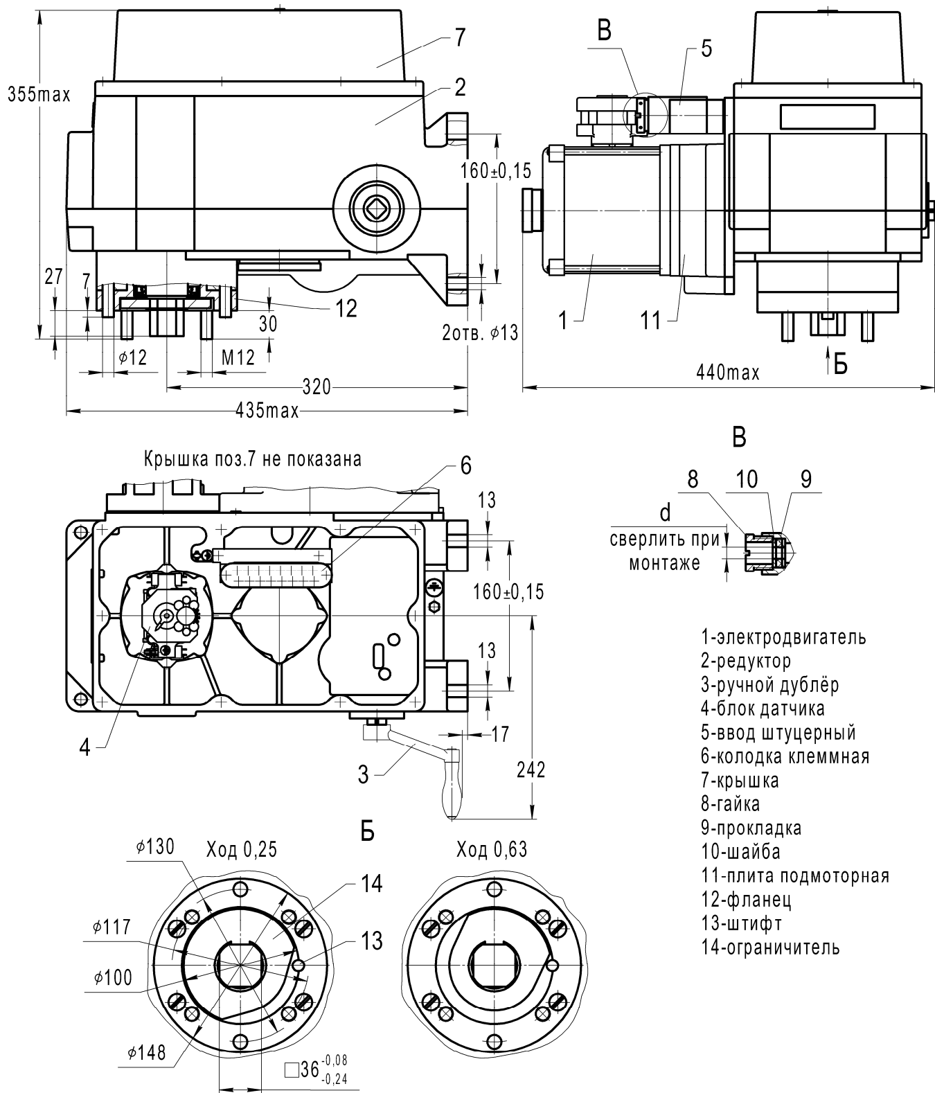
Рис.А.3 МЭО-630, -1000-ИСТ4-93 (на лапах)
