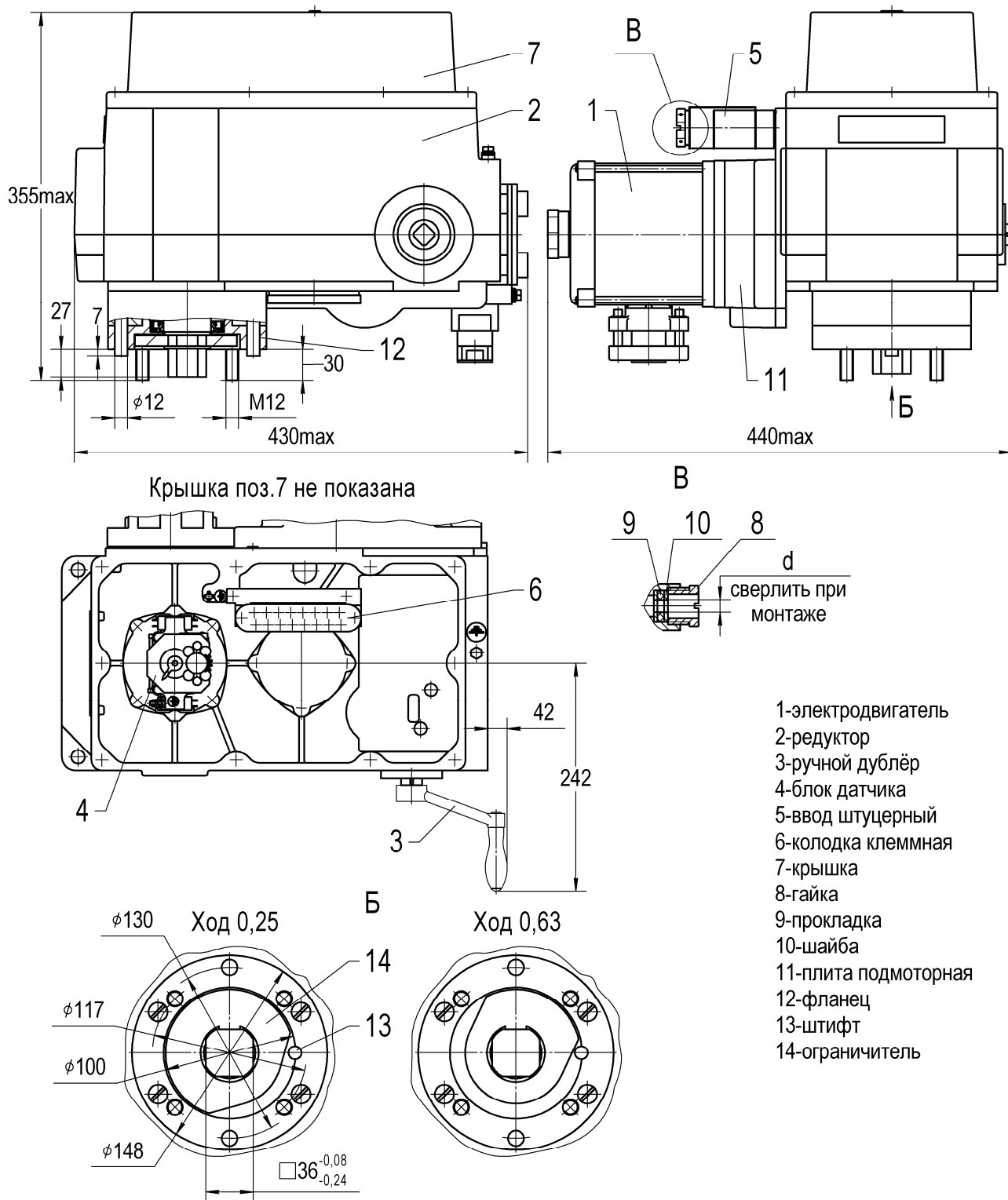
Рис.А.1 МЗО-630, -1000-ICT4-93
