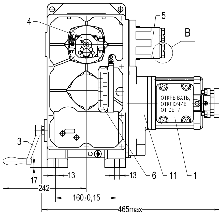
Рис.А.2 МЭО-630, -1000-ИСТ4-95
