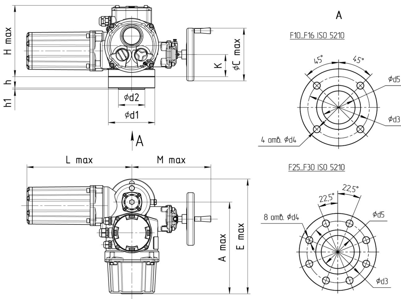
Рис.Б1 Габаритные и присоединительные размеры механизмов МЭМ15.3
