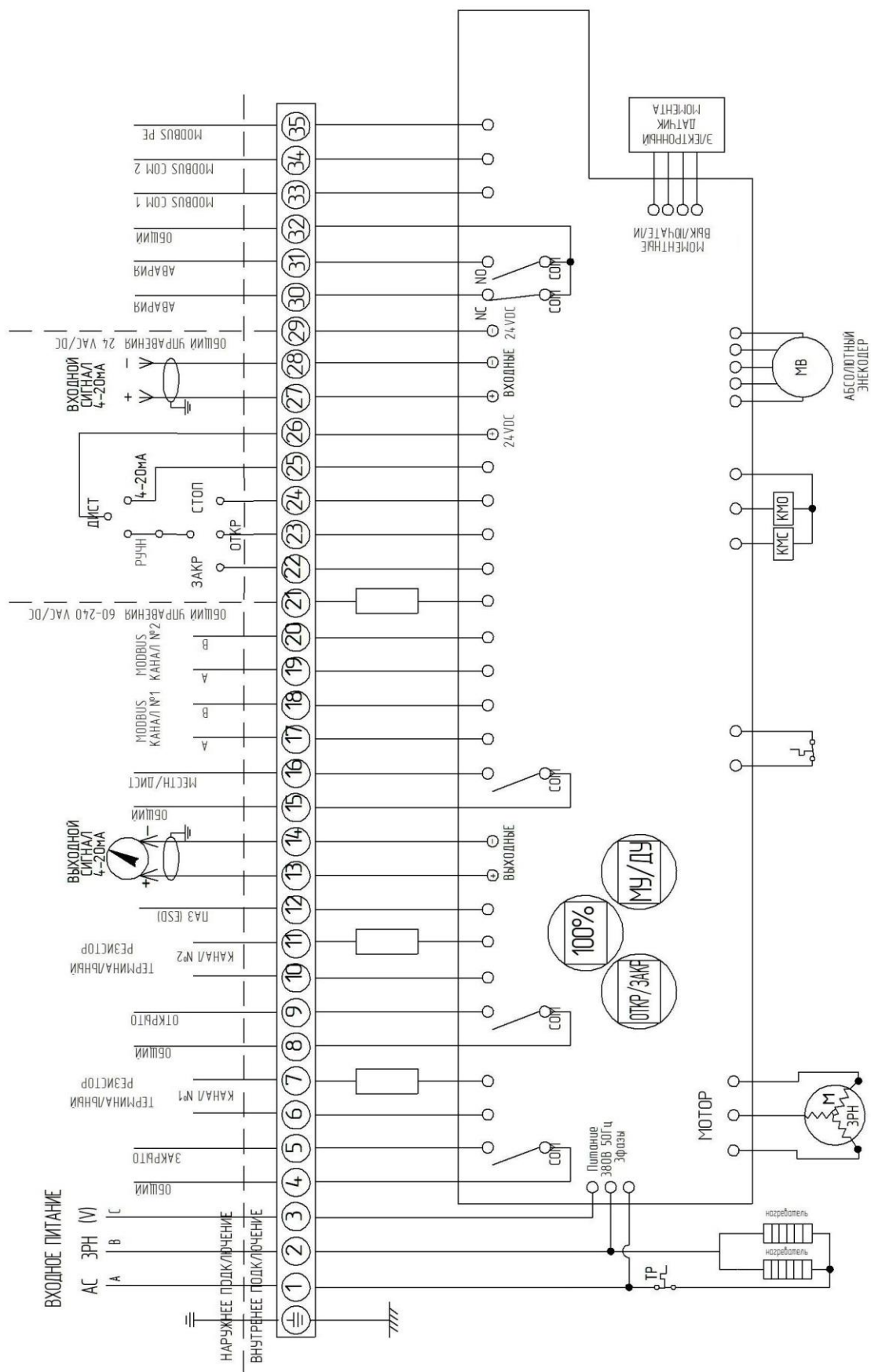
Рисунок В.6 - Схема принципиальная С22, С23 для механизма 380В с цифровым протоколом Modbus (1 канал с резервом)
